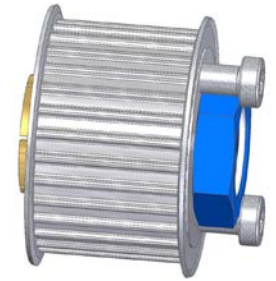
Abb.: 13 Kegelhemmung gelöst, BG kann entfernt werden
