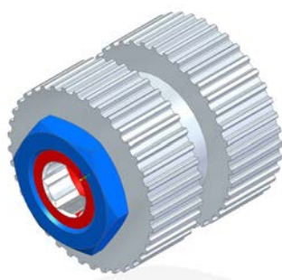
Abb.: 3 Die Darstellung - rechts in der Schnittrichtung - zeigt eine solche, vom Kunden vorgegebene Zahnriemenscheibe. Die Ausführung beinhaltet das BOQA® Befestigungselement, sowie die Befestigungsmutter.
