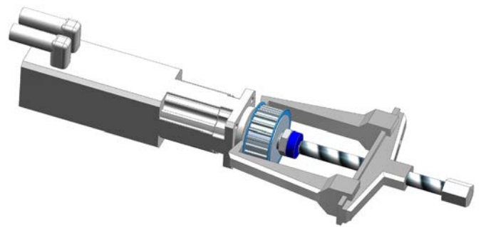
Abb.: 8 Darstellung des Abziehvorganges (Lösen der Kegelhemmung des BOQA® Befestigungselements mit einem gebräuchlichen Klauenabzieherwerkzeug
