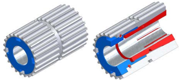
Abb.: 4 Darstellung der Ausführung einer extrem platzsparenden Befestigung mit dem BOQA® Befestigungselement mit integrierter Abdrückeinrichtung zur Lösung der Kegelhemmung.
