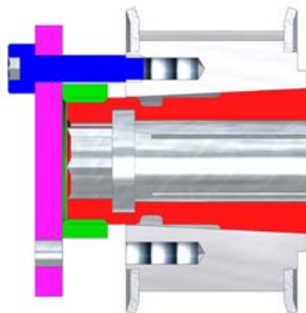
Abb.: 15 Erste Abdrückschraube mit Abdrückplatte platziert
