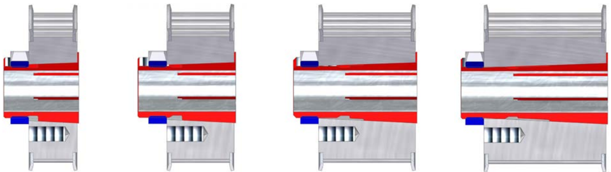
Abb.: 2 Darstellung der unterschiedlichen Nabenbreiten, die mit Standardausführungen des BOQA® Befestigungselements auf Wellen befestigt werden können, am Beispiel der GRUPPE 2350
