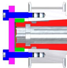
Abb.: 16 Zweite Abdrückschraube platziert
