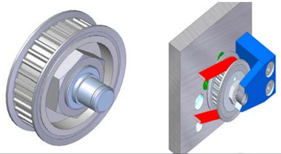
Abb.: 5 Darstellung unterschiedlicher Ausführungen der Gegenlagerung mit BOQA® Befestigungselementen mit integriertem Gegenlagerzapfen.
