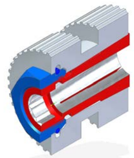
Abb.: 3 Die Darstellung - rechts in der Schnittrichtung - zeigt eine solche, vom Kunden vorgegebene Zahnriemenscheibe. Die Ausführung beinhaltet das BOQA® Befestigungselement, sowie die Befestigungsmutter.
