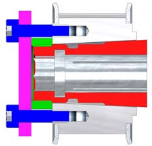
Abb.: 17 Kegelhemmung gelöst, BG kann entfernt werden
