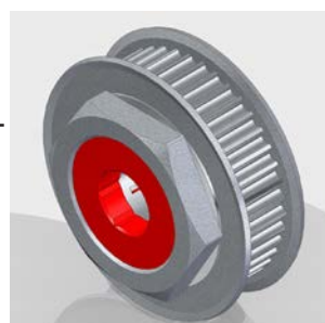
Abb.: 18 Zahnscheiben-BG m. integr. Abdrückeinrichtung
