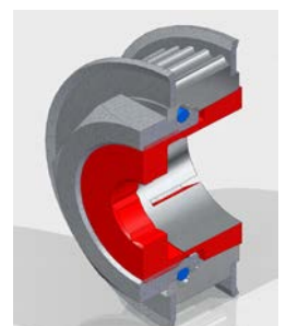
Abb.: 19 Zahnscheiben-BG (Schnitt)
