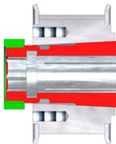
Abb.: 14 Befestigungsmutter um 2 - 3 Umdrehungen gelöst
